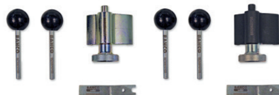
▶ BE509205 JUEGO DE CALADO GRUPO VAG DIESEL 1.6, 1.9, 2.0 (UTIL CIGÜENAL REDONDO) • Audi, Seat, Skoda, Volkswagen • Motores 1.6TDI CR, 1.9TDI, 2.0TDI CR
